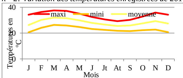
Figure n° 2: Variation des températures enregistrées de 2010 à 2015
