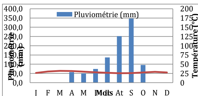
Figure n° 3 : Diagramme ombrothermique de Mango (20117)
